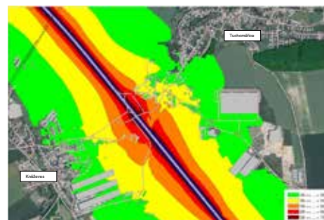
Hluková mapa ve výšce 4 m nad terémem – denní doba
